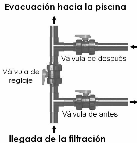
Esquema By-pass
