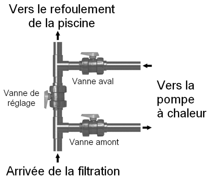
Schéma du by-pass
